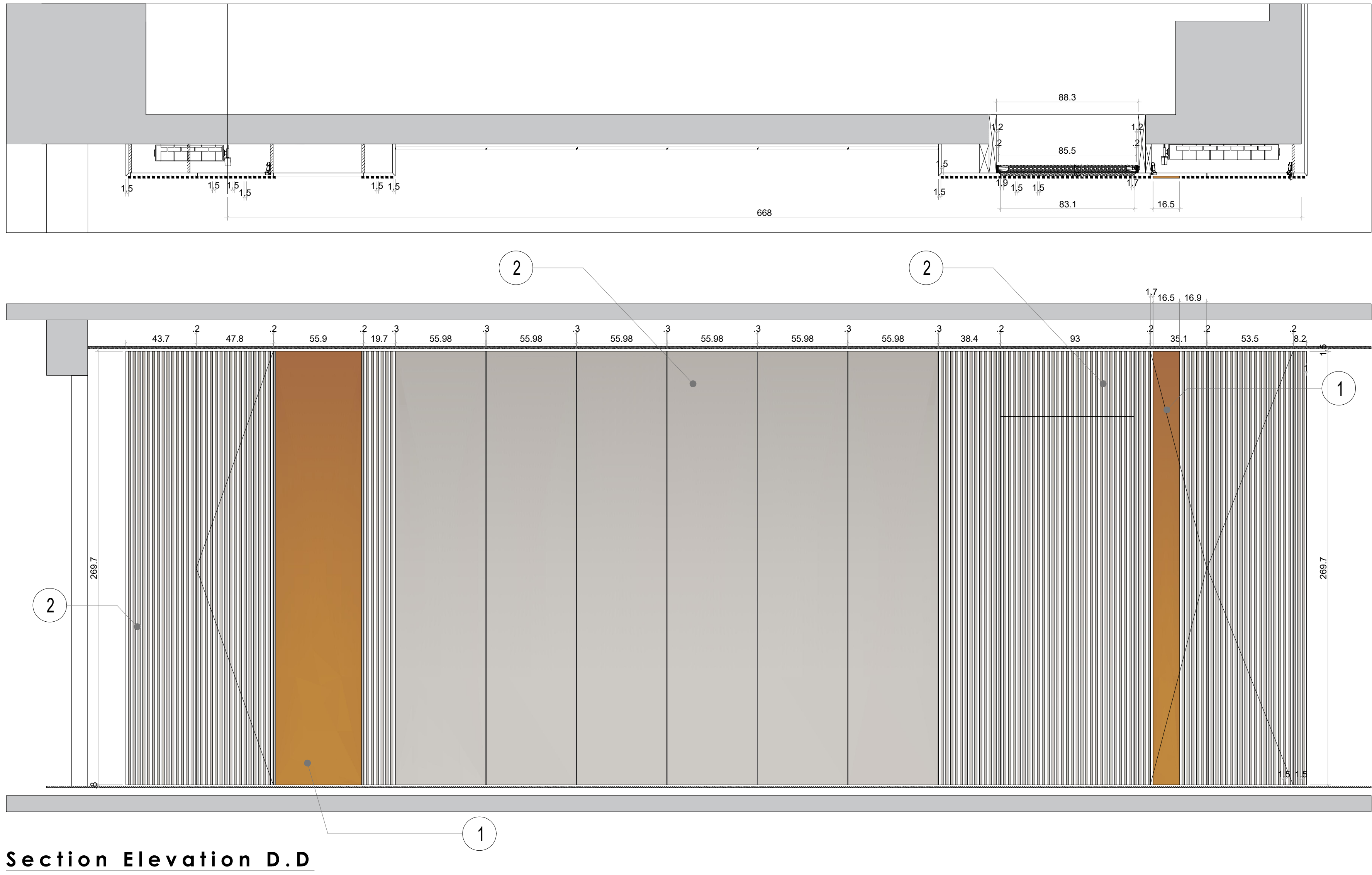
Section Elevation D.D
