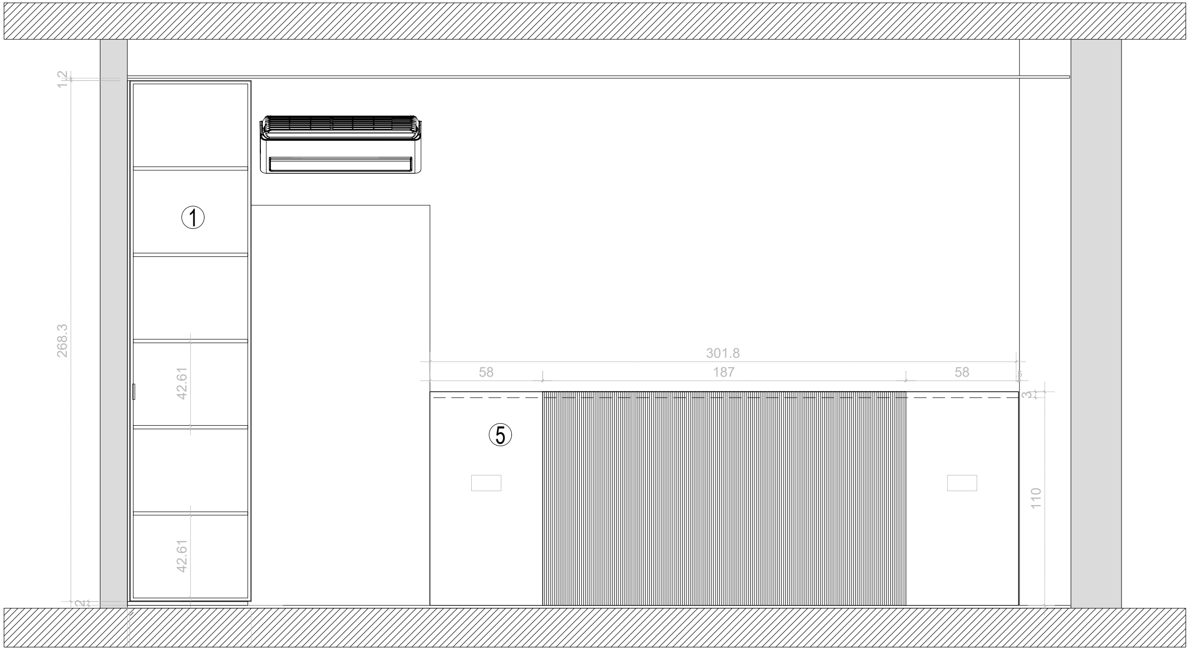
Section Elevation B.B
