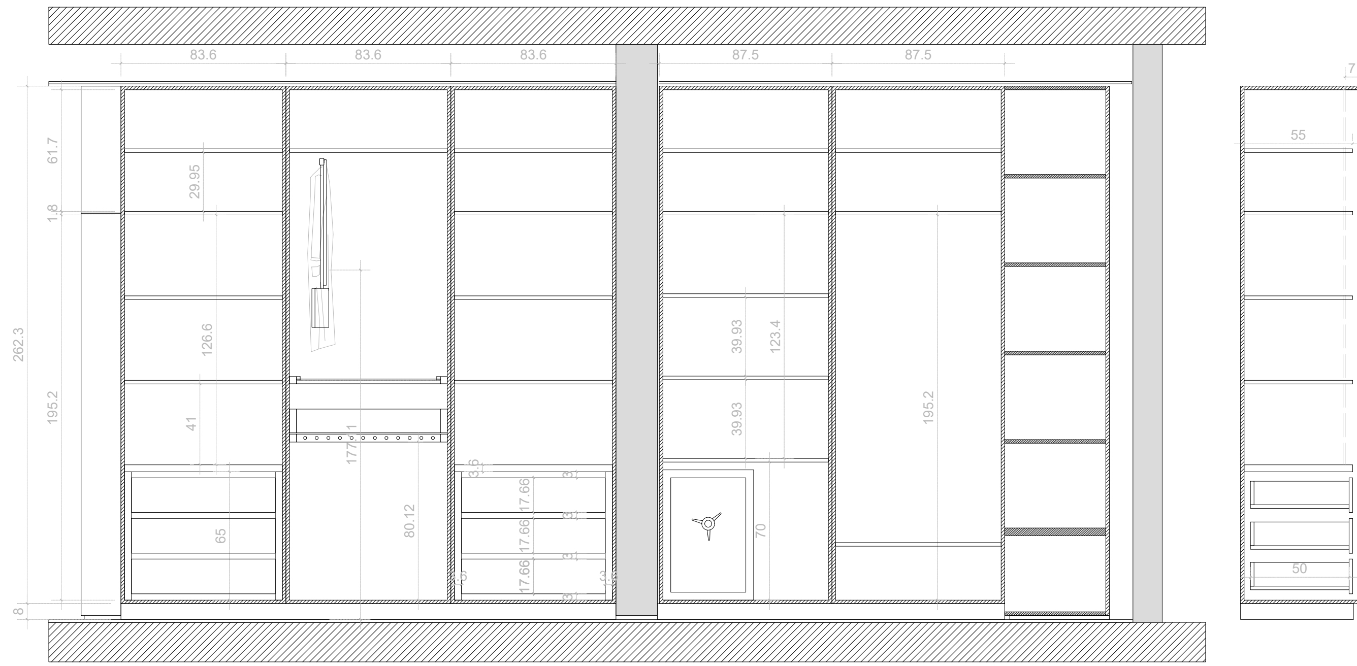
Section Elevation A.A
