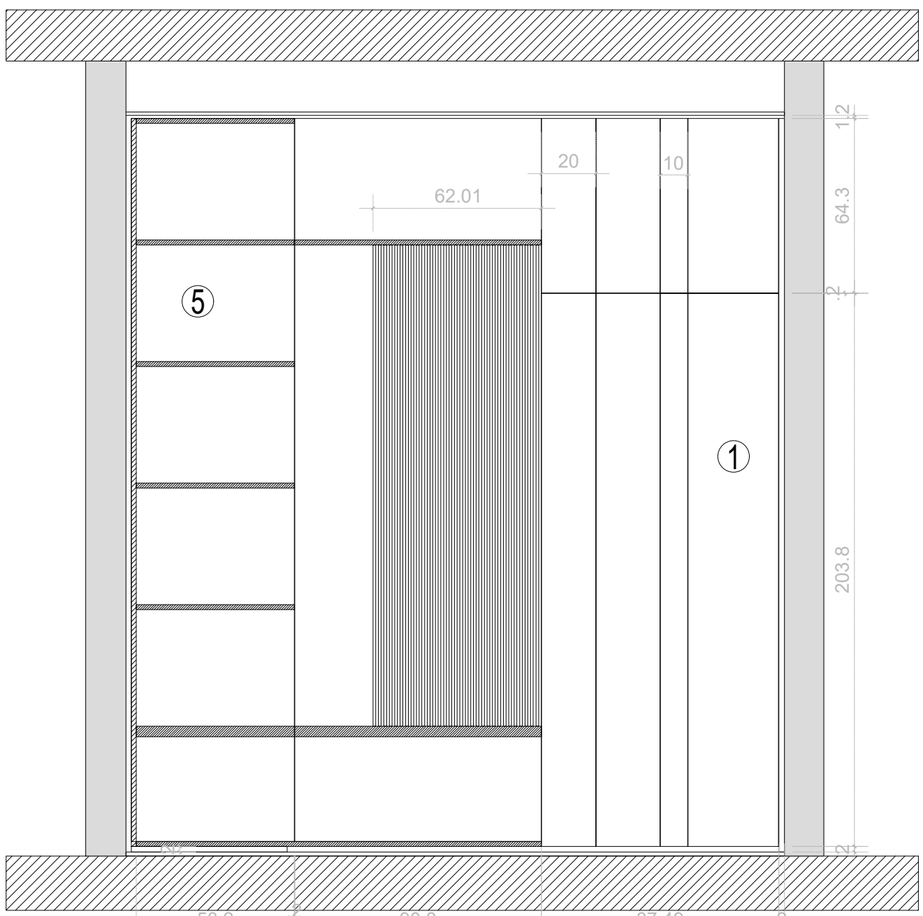
Section Elevation D.D
